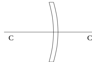
3- Ménisque divergent
